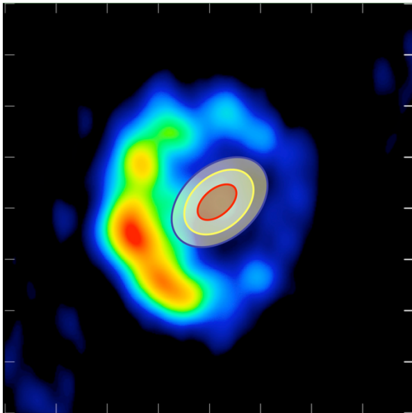
Imagen de interferometría y ondas de radio de RS Ophiuchi obtenida días después de su estallido de 2006.
