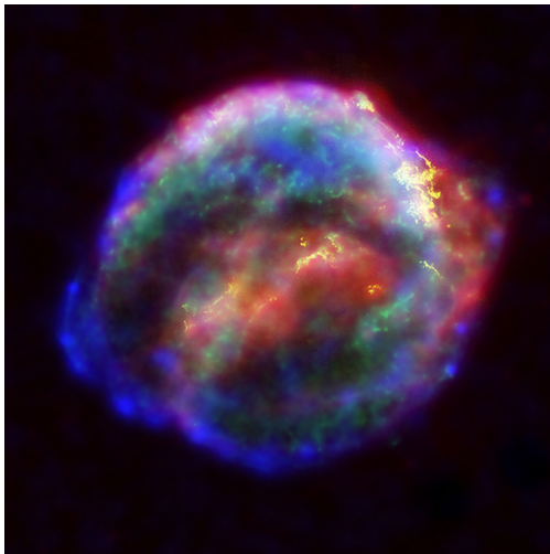
Resto de la supernova de Kepler, cuya luz llegó a la Tierra en 1604.
