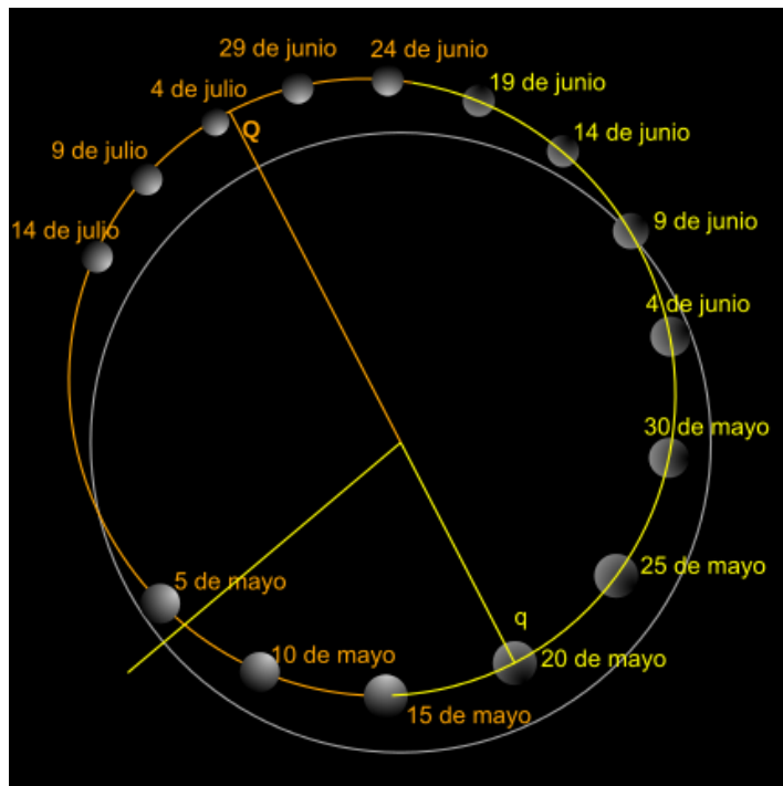
Órbita de Mercurio (en amarillo)
